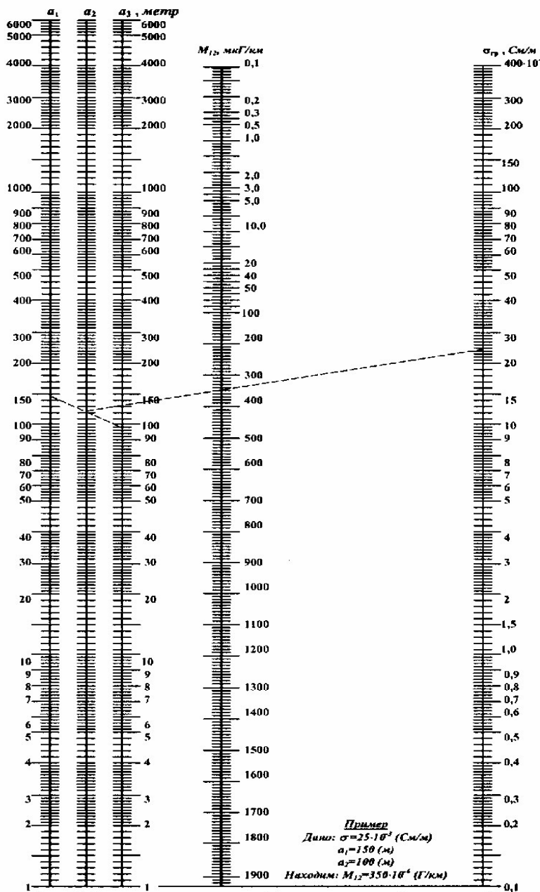
Рис. 6.2. Номограмма расчета коэффициента взаимной индукции M_{12}
