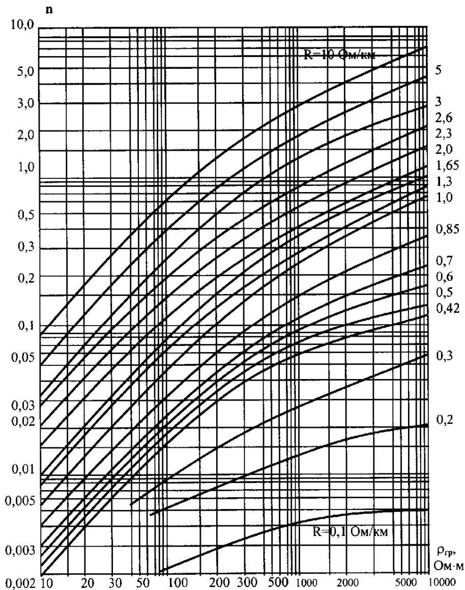
Рис. 6.3 Графики вероятного числа повреждений n кабеля связи от ударов молнии
